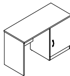
СТОЛ С ПРАВОЙ ТУМБОЙ ПОД ФРИГОВАР (VG410DX) Ш: 1200 / Г: 520 / В: 750
