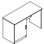
СТОЛ С ЛЕВОЙ ТУМБОЙ ПОД ФРИГОВАР (VG410SX) Ш: 1200 / Г: 520 / В: 750
