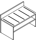
ТУМБА БАГАЖНАЯ (VG340) Ш: 900 / Г: 520 / В: 587
